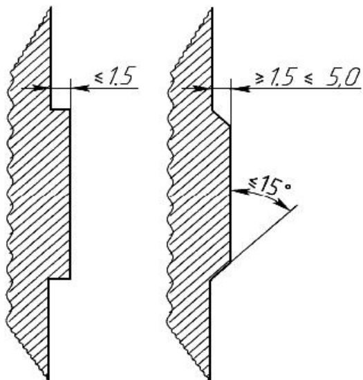
Рисунок 11 - Размеры допустимых выступов в зонах перемещения
