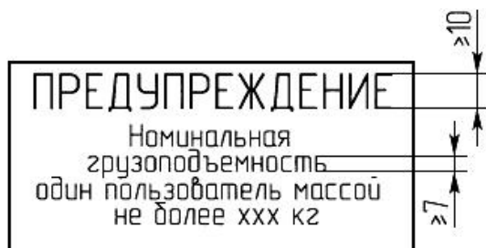
Рисунок 15 - Образец стандартной надписи с информацией о грузоподъемности
