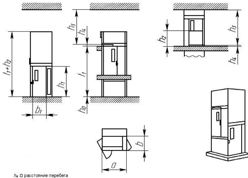
Рисунок 6 - Подъемная платформа с огражденной зоной перемещения
